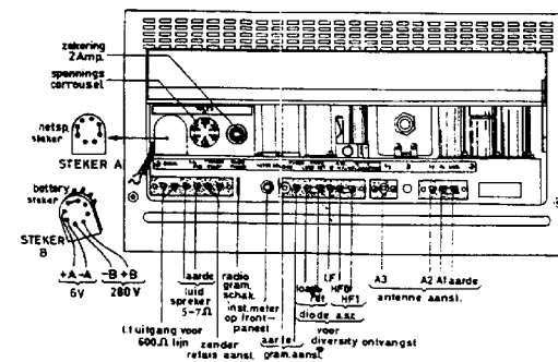
FIG. 9 ACHTERAANZICHT
