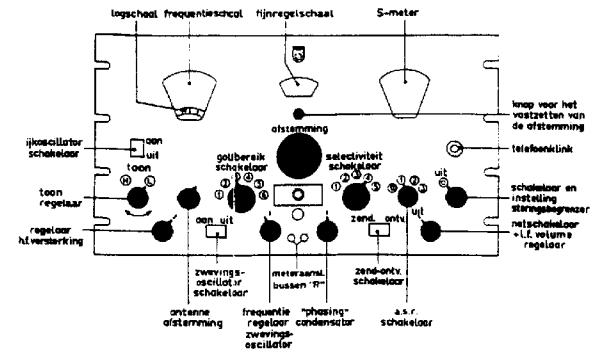
FIG. 8 VOORAANZICHT
